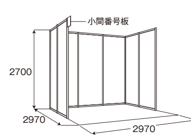
■ 立面図 (例：1小間)
